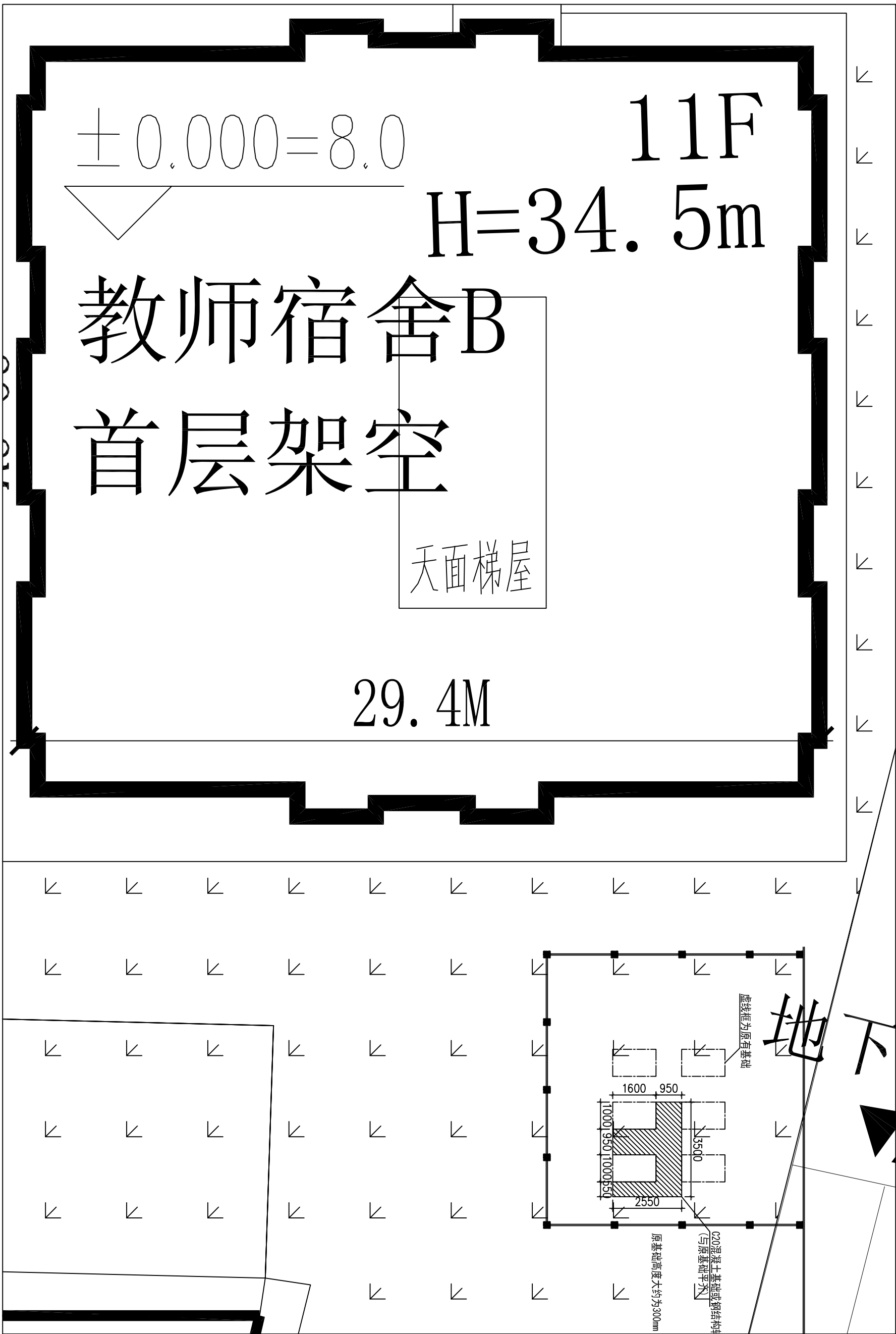
广大教B地面设备基础图 1:100
