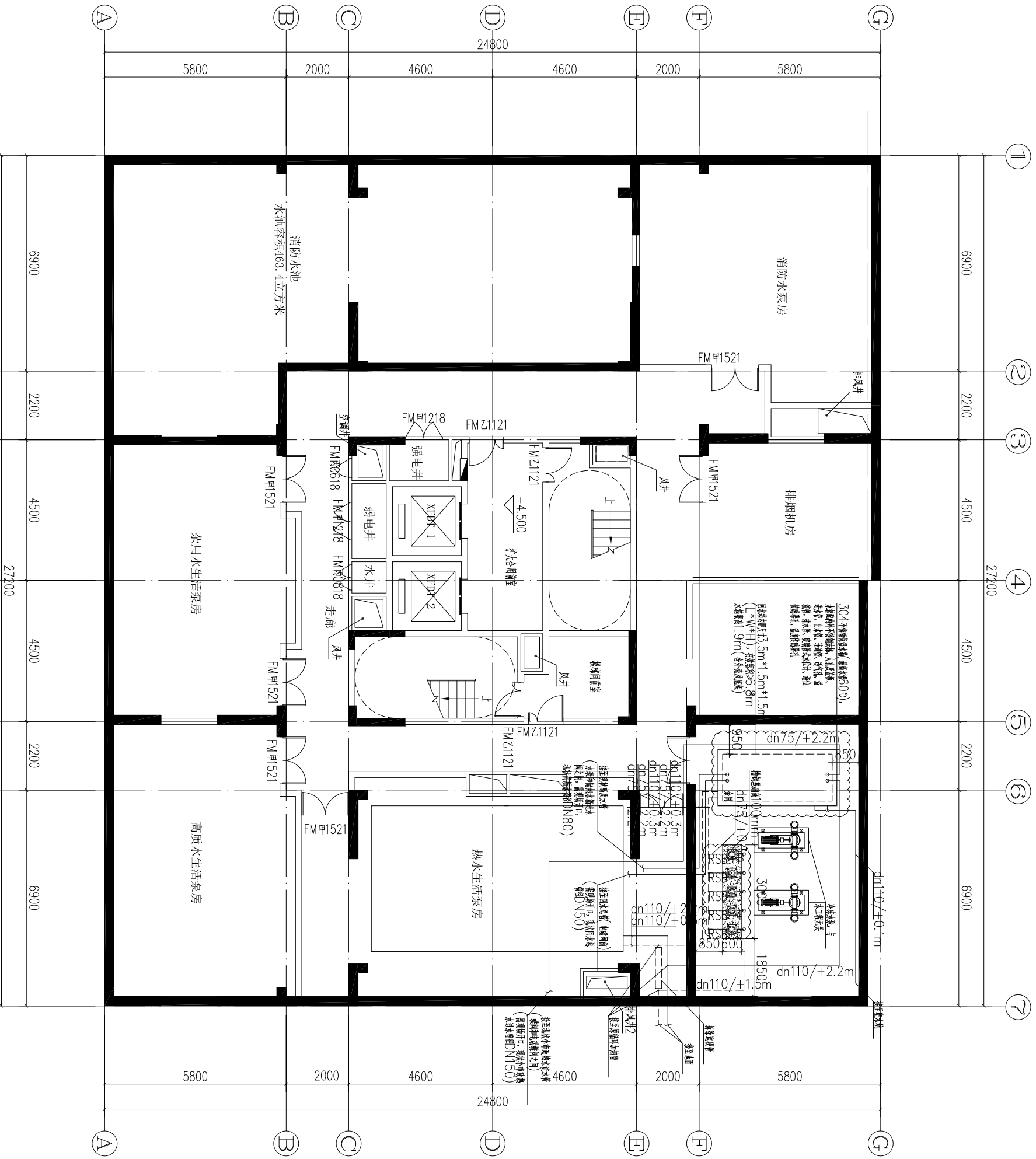
负一层制热平面图
